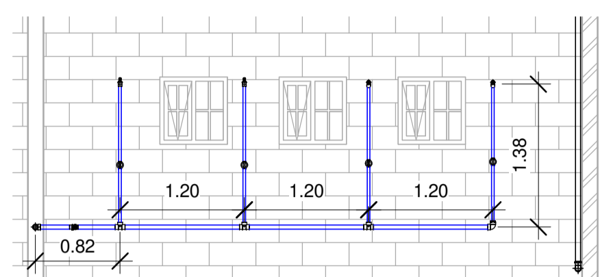
2 (cotas) 1:50
