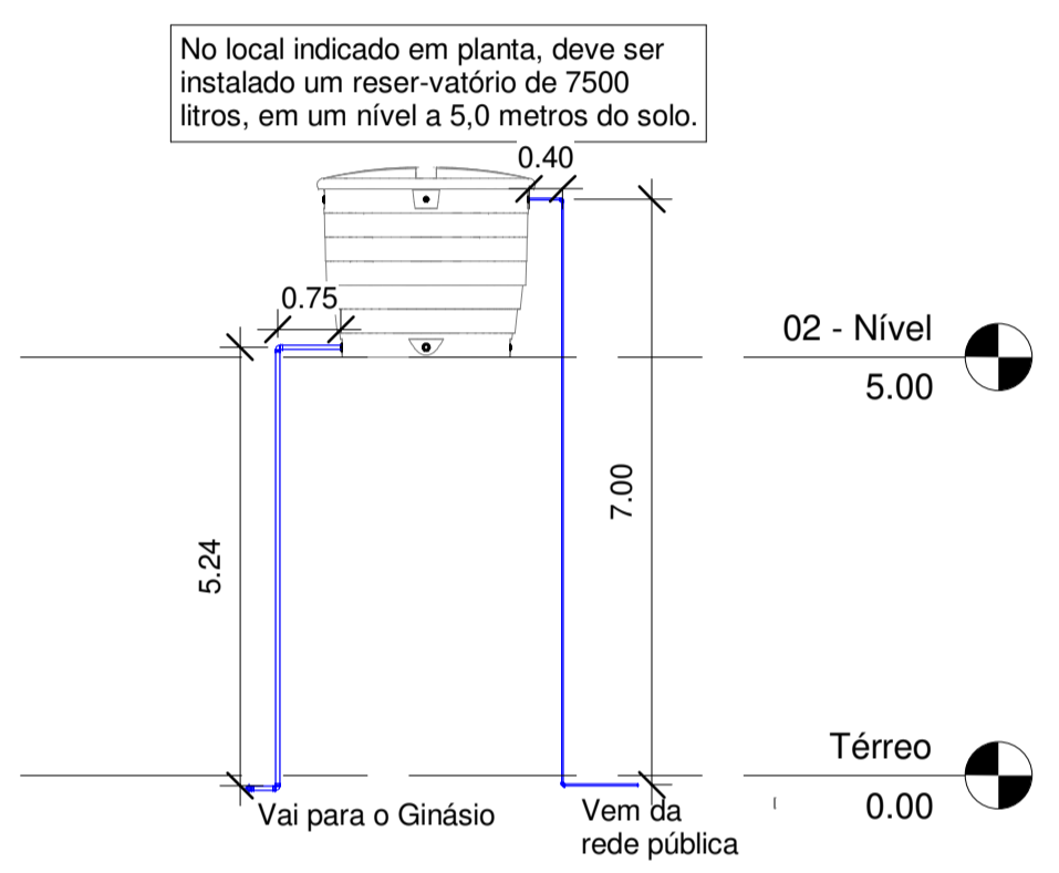
3 (cotas) 1:100
