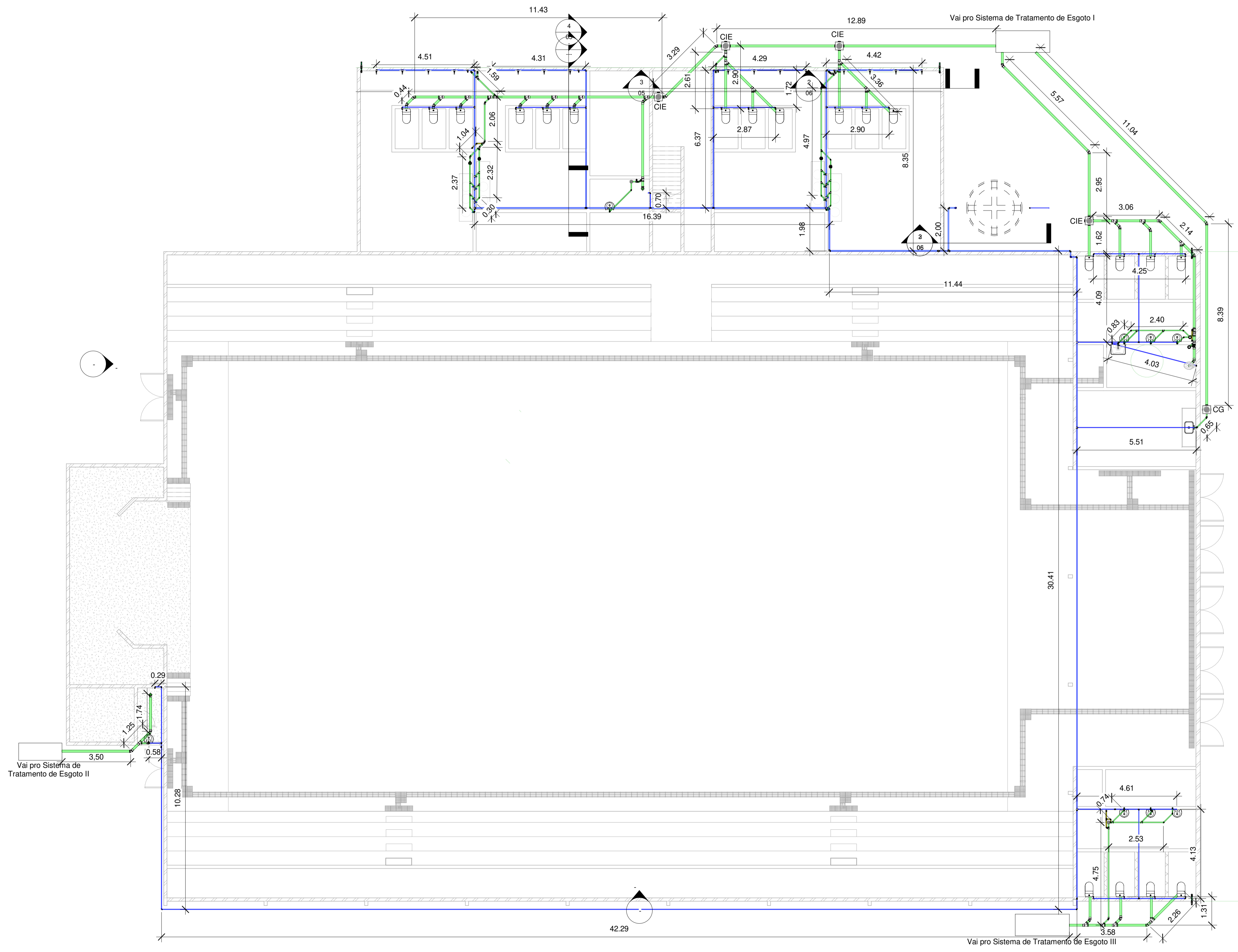
1 Hidrossanitário 1:100
